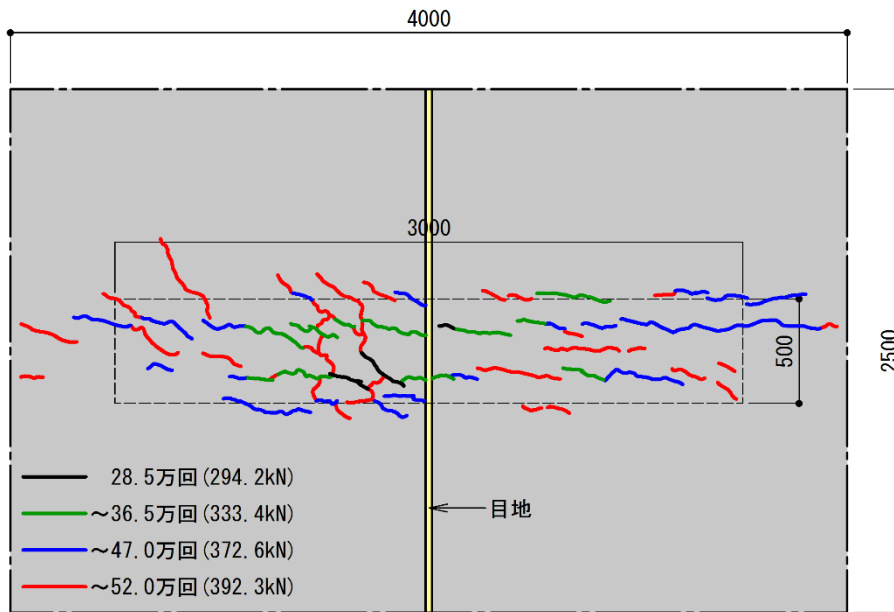
【床版下面のひび割れ状況】
